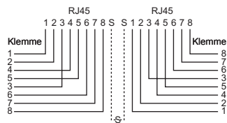
Schema c8
